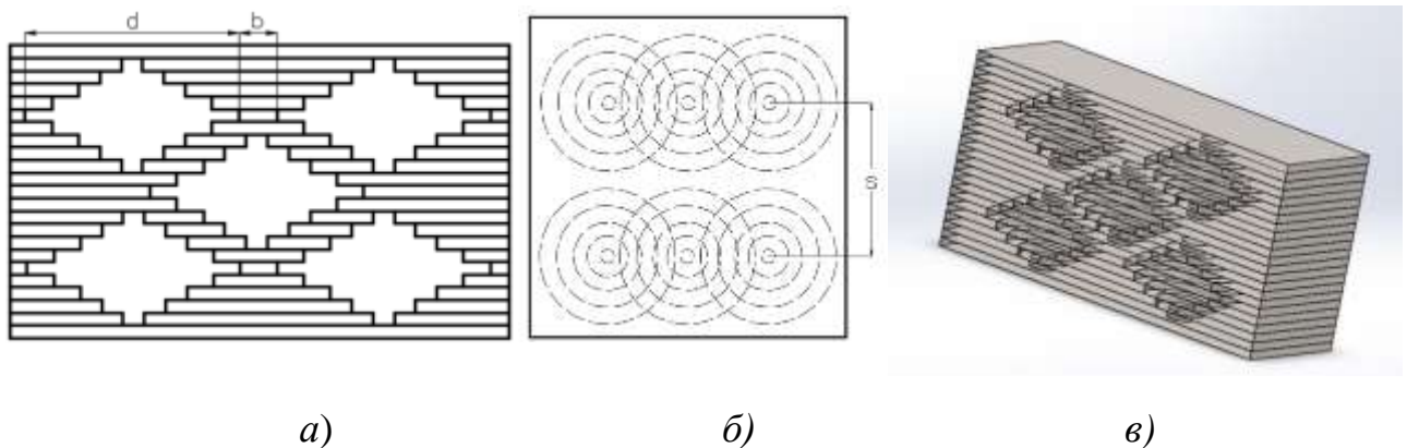
Рис. 17. Зібрані металеві перфоровані пластини: вид збоку (а); вид зверху (б); аксонометричний розріз комп'ютерної тривимірної моделі (в)
