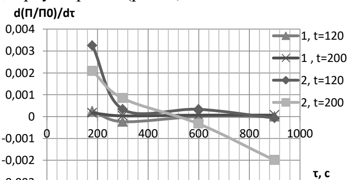
Рис. 3. Динаміка зміни пористості в вогнетривкій суміші
