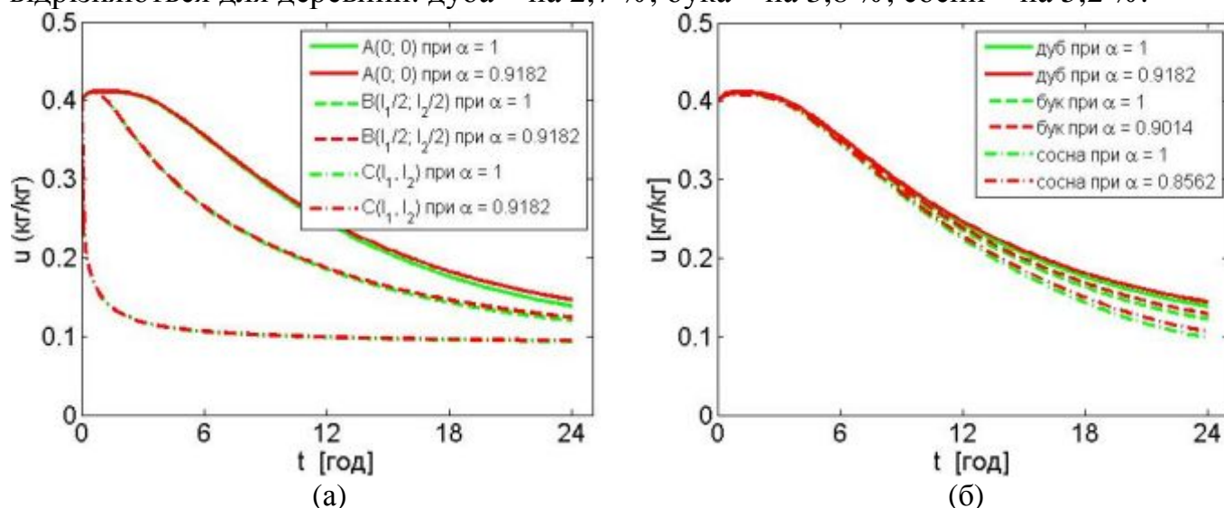
Рис. 2. Зміна вологовмісту у точках A(0;0) , B(l_1/2; l_2/2) і C(l_1; l_2) поперечного перерізу дубового бруска (а) та у точці C(l_1; l_2) (б) для брусків із різних порід деревини
