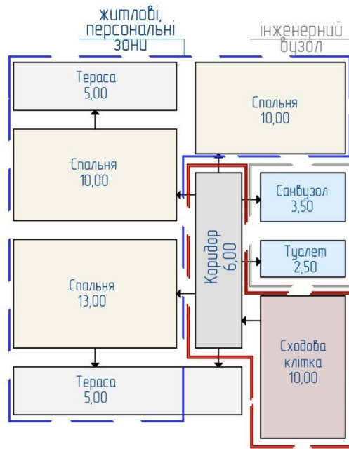
Рис. 9. Архітектурно-планувальна структура котеджу для проживання однієї невеликої групи відпочивальників (рисунок автора).
