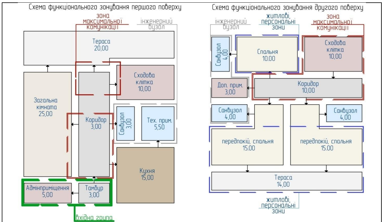
Рис. 10. Архітектурно-планувальна структура котеджу готельного типу (рисунок автора).
