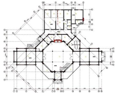
Ресторан "Villa park" в с.Підпечери, Тисменицького р-ну, Івано-Франківської обл.
