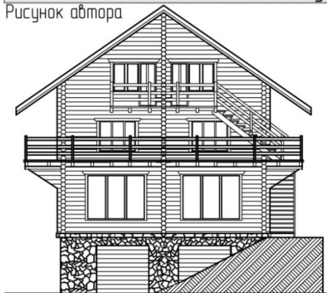
Рис. 8. Типи котеджів із зовнішніми вертикальними та горизонтальними комунікаціями (рисунок автора).
