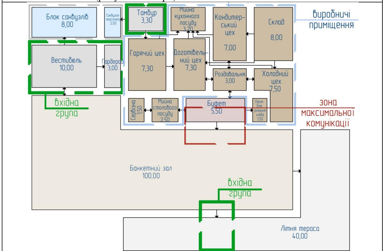
Рис. 5. Архітектурно-планувальна структура кафе-ресторану, що входить в структуру відпочинкового комплексу (рисунок автора).
