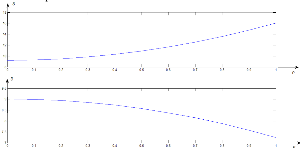
Рис.3. Графік розподілу мас порядку в точці \varphi = 60^0 , \lambda = 0^0 по радіусу для однорідної моделі та моделі PREM.
