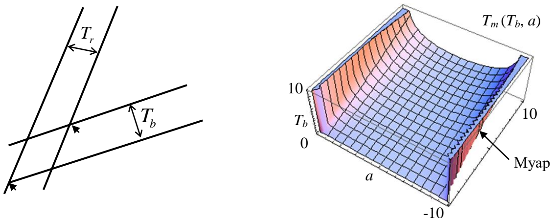
Рисунок 5 – Схема залежності періоду зміни муарної решітки T_m від кута нахилу решітки базового шару \alpha_b та періоду базового шару T_b \in [0 \dots 0,01]
