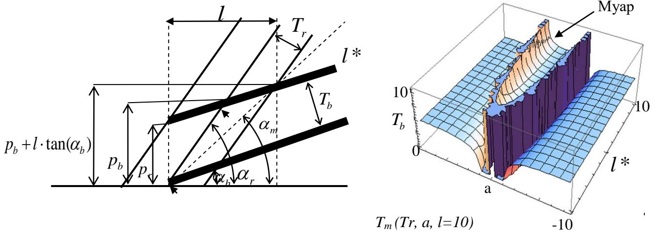
Рисунок 7 – Схема залежності періоду зміни муарної решітки T_m від кута нахилу решітки базового шару \alpha_b та періоду базового шару T_r \in [0 \dots 0,01]
