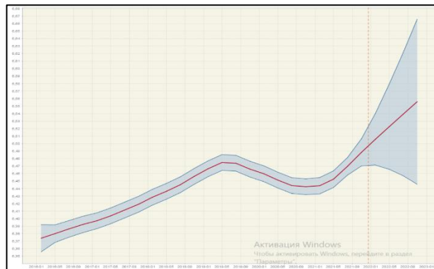
Рис. 3. Лінія тренду ВВП в постійних цінах 2016 року в програмі «JDemetra+»
